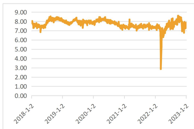
图 1.35: 沪伦比值
