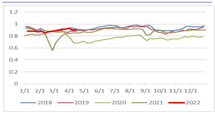
图 4：EIA 美国炼厂开工率：%
