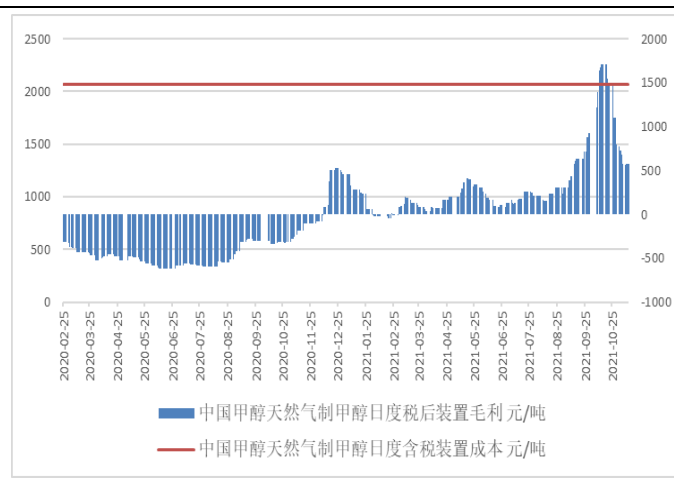
图 4：天然气制甲醇现金流
