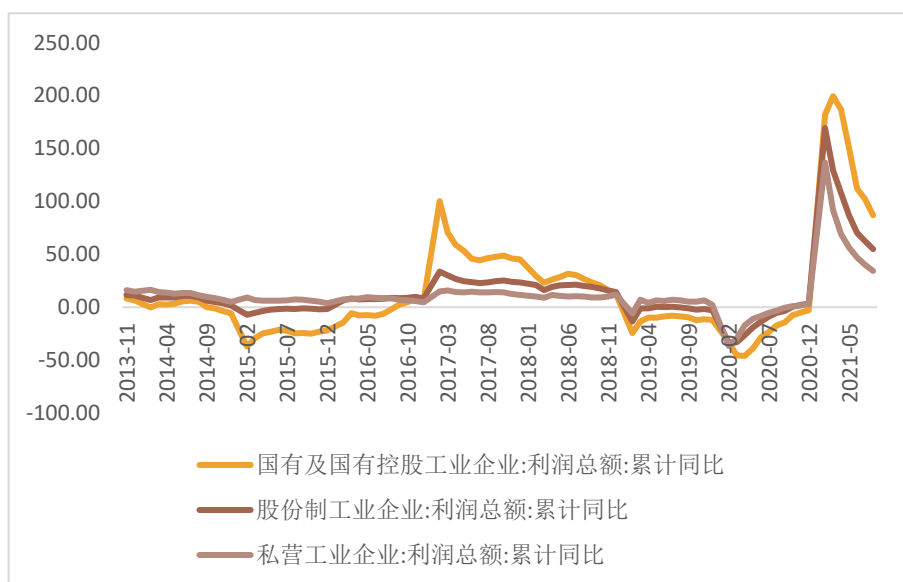
图 3：不同所有制企业利润累计同比：单位：%
