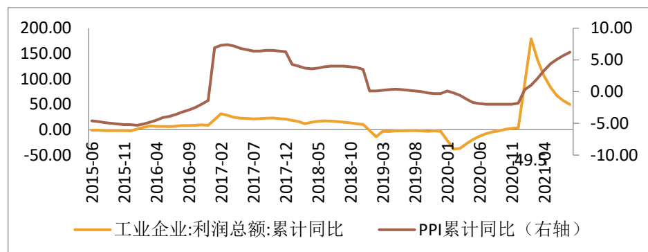
图 1：企业利润累计同比：单位：%
